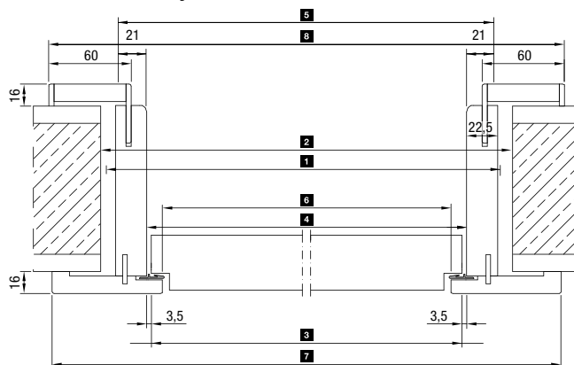
Horizontálne rezy
