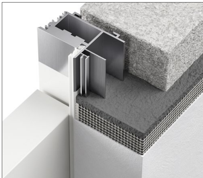
Dodatočná flexibilná tkanina zabraňuje tvorbe prasklín v omietke.
